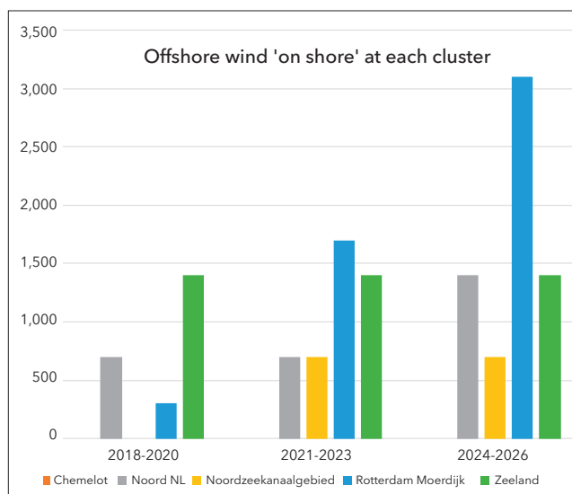
Figuur 3 - Match in geografie en vermogen van P2H potentieel met offshore wind aanlanding 2
